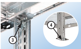
Fachbodenträger (3), Klemmfuß (4)
